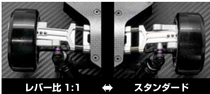
新設計の非対称ナックル
